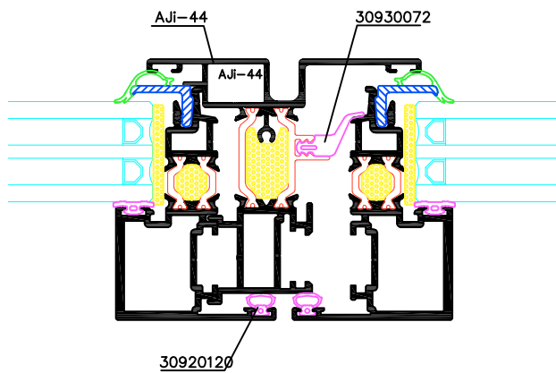
Secção central (corte 2)
