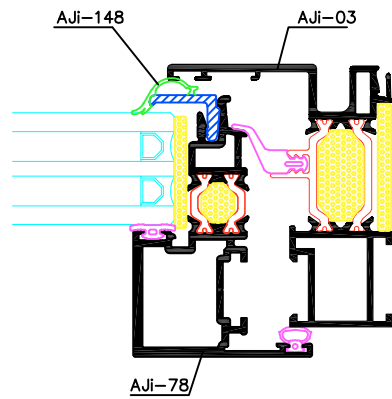
Secção lateral (corte 1)
