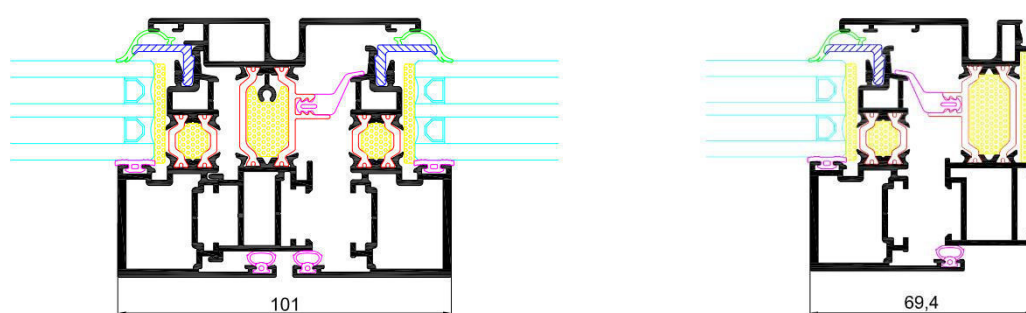
Secção central (corte 2)
