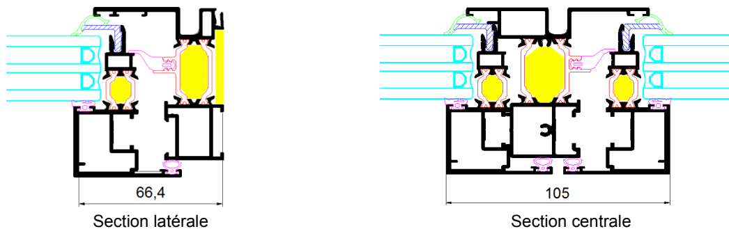
Figure 1: Représentant des profilés de fenêtre Système AJi – Ouvrant Caché Rainure 16 de l'Anicolor (dimensions en mm).
