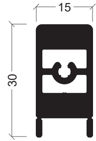
KL-87 Perfil de reforço Refuerzo
