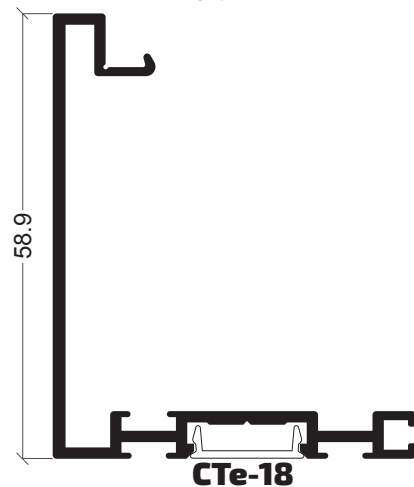
CTe-18 Tampa cruzamento recta Tope cruzamiento recta
