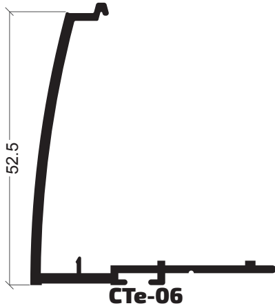
CTe-06 Tampa cruzamento Tope cruzamiento
