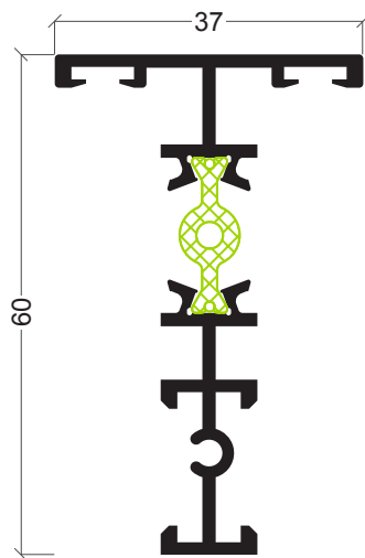
ARi-40 Divisor de vidro
