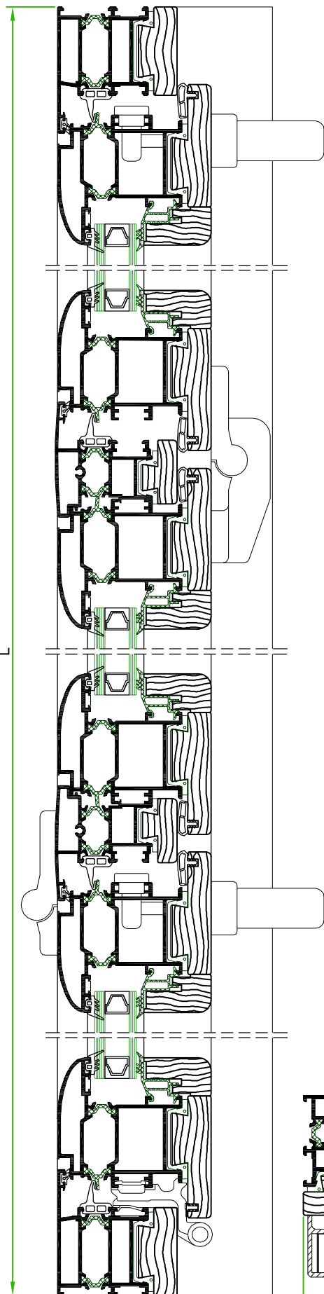
SECÇÃO A - A
