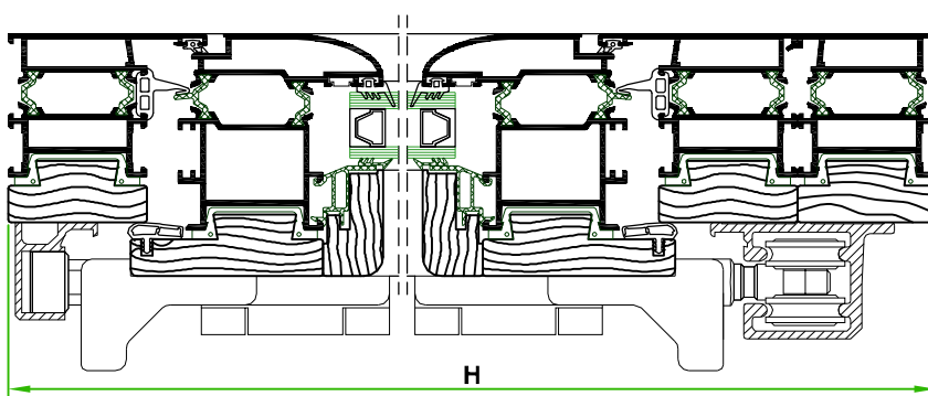
SECÇÃO B - B
