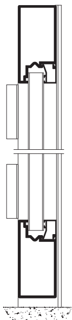
Secção A-A
