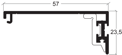
CW-26 Tampa de cruzamento CW minimal Tope de cruce CW minimal
