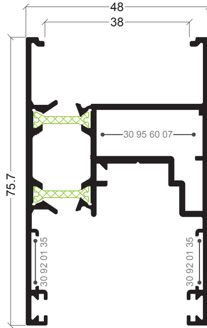
CW-03 Aro móvel perimetral Hoja perimetral
