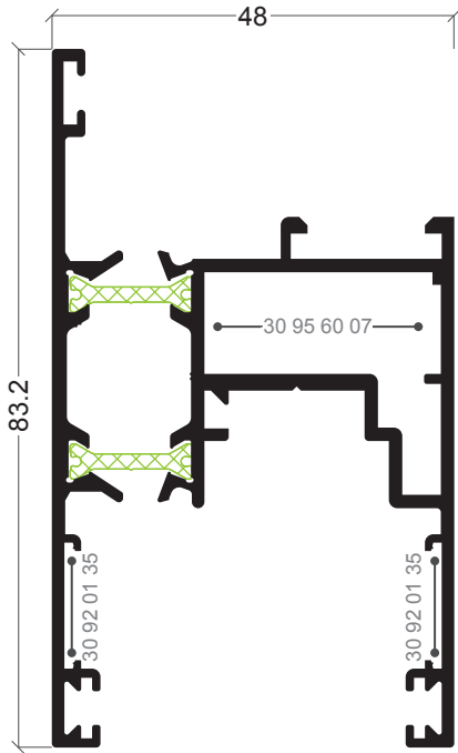
CW-02 Aro móvel perimetral Hoja perimetral
