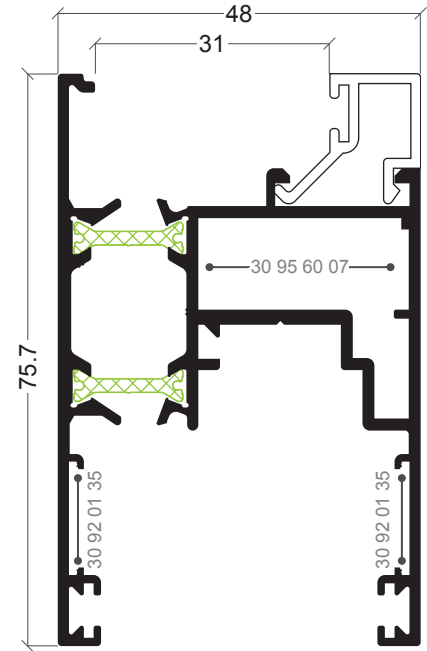
CW-04 Aro móvel perimetral Hoja perimetral
